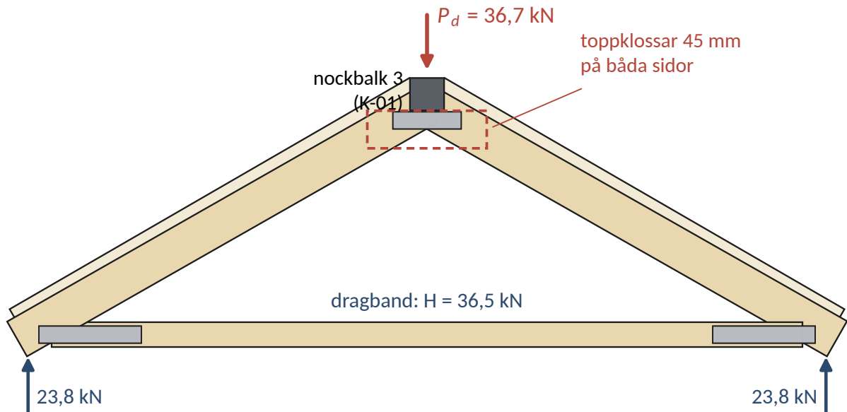
Figur 3: Mittakstolen L2M i elevation ur modellen, med last och krafter. Gaveltakstolarna har samma form men bär mindre.
