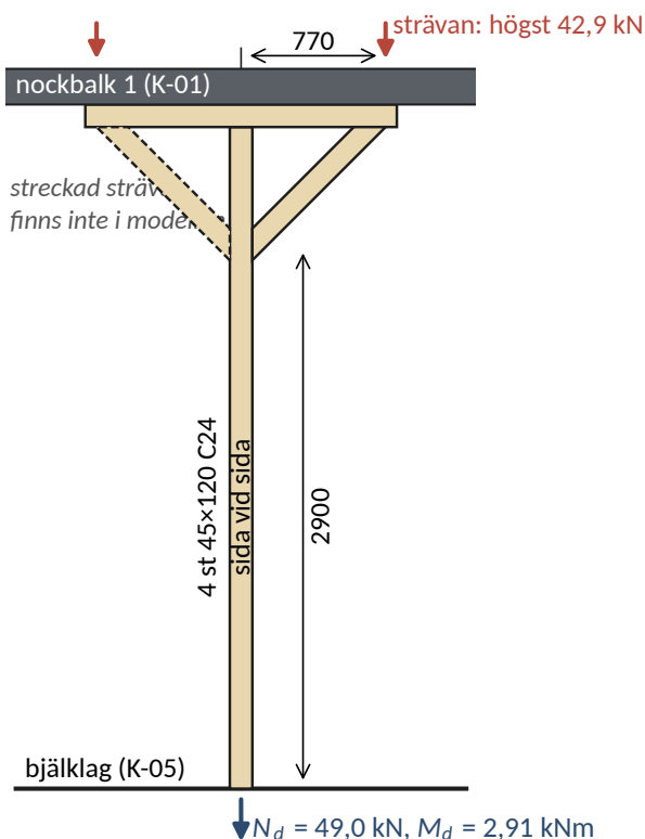
Figur 4: Huvudstolpen under nockbalk 1, stöd D. Strävor på båda sidor.
