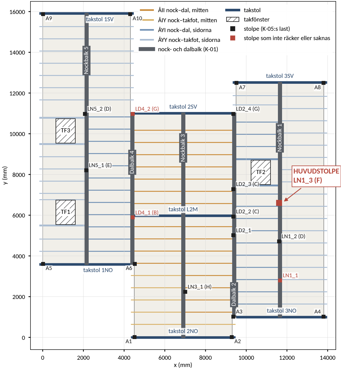
Figur 1: Takets bärande delar i plan, koordinater som i K-05. Röda stolpar räcker inte eller saknas i modellen, se tabellen nedan.
