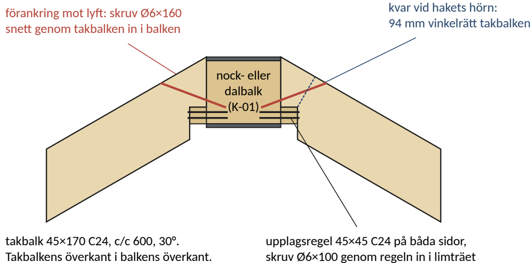
Figur 2: Takbalkarnas upplag motnockbalken, snitt tvärs balken. Vid dalbalken på samma sätt, spegelvänt.
